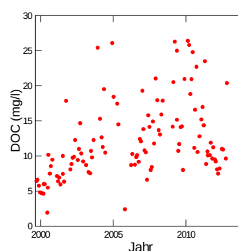
Abb. 284 Entwicklung der Chloridkonzentration (links) und der Konzentration an gelöstem organischem Kohlenstoff (rechts) in der Bodenlösung der Fichtenbeobachtungsfläche Sagno in 60 cm Tiefe
