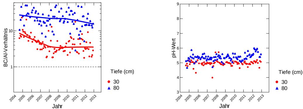
Abb. 121: Entwicklung des BC/Al-Verhältnisses (links) und des pH-Wertes (rechts) in der Bodenlösung der Fichtenbeobachtungsfläche Busswil.
