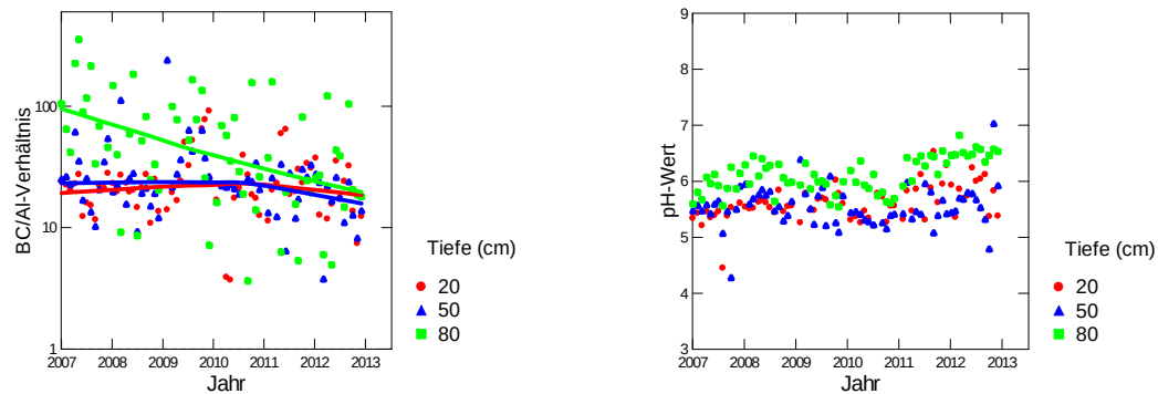
Abb. 169: Entwicklung des BC/Al-Verhältnisses (links) und des pH-Wertes (rechts) in der Bodenlösung der Fichtenbeobachtungsfläche Le Châtelard.
