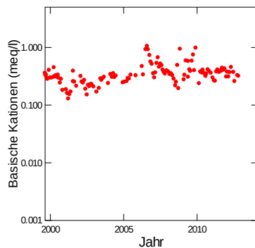
Abb. 282: Entwicklung der Konzentration von basischen Kationen (BC) (links) und der Konzentration von anorganischem Aluminium (rechts) in der Bodenlösung der Fichtenbeobachtungsfläche Sagno in 60 cm Tiefe. Die gestrichelte Linie in der rechten Grafik ist die kritische Al-Konzentration.
