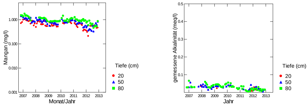
Abb. 133: Entwicklung der Mangankonzentration (links) und der gemessenen Alkalinität (rechts) in der Bodenlösung der Fichtenbeobachtungsfläche Diessenhofen.
