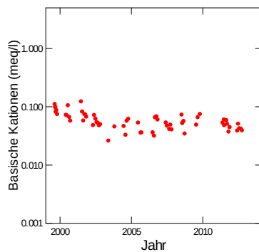
Abb. 178: Entwicklung der Konzentration von basischen Kationen (BC) (links) und der Konzentration von anorganischem Aluminium (rechts) in der Bodenlösung der Fichtenbeobachtungsfläche Lurengo in 60 cm Bodentiefe. Die gestrichelte Linie in der rechten Grafik ist die kritische Al-Konzentration.
