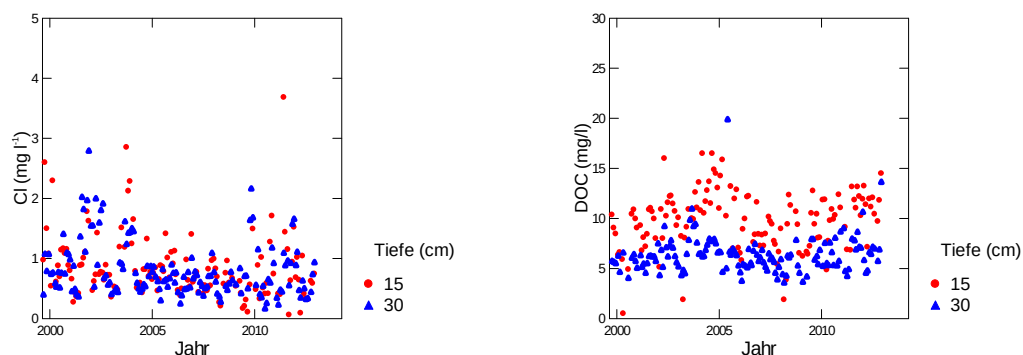
Abb. 148: Entwicklung der Chloridkonzentration (links) und der Konzentration an gelöstem organischen Kohlenstoff (rechts) in der Bodenlösung der Beobachtungsfläche Grenchenberg (Buchen/Fichten).
