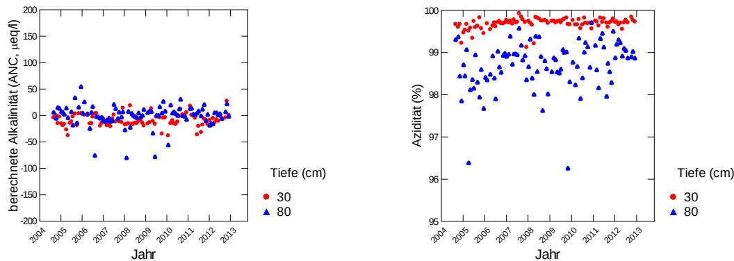
Abb. 126: Entwicklung der berechneten Alkalinität (links) und der Azidität (rechts) in der Bodenlösung der Fichtenbeobachtungsfläche Busswil.
