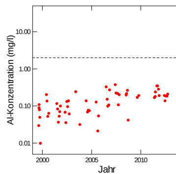
Abb. 178: Entwicklung der Konzentration von basischen Kationen (BC) (links) und der Konzentration von anorganischem Aluminium (rechts) in der Bodenlösung der Fichtenbeobachtungsfläche Lurengo in 60 cm Bodentiefe. Die gestrichelte Linie in der rechten Grafik ist die kritische Al-Konzentration.
