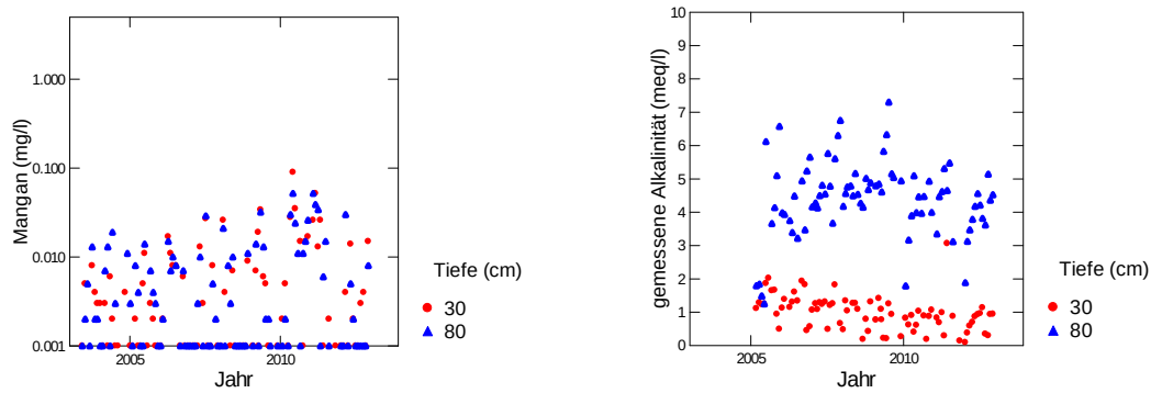
Abb. 317: Entwicklung der Mangankonzentration (links) und der gemessenen Alkalinität (rechts) in der Bodenlösung der Fichtenbeobachtungsfläche Winterthur
