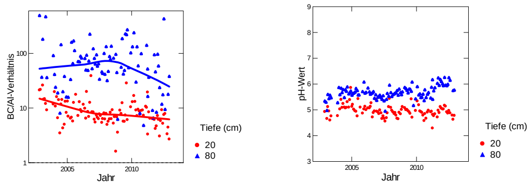
Abb. 33: Entwicklung des BC/Al-Verhältnisses (links) und des pH-Wertes (rechts) in der Bodenlösung der Buchenbeobachtungsfläche Aarwangen.
