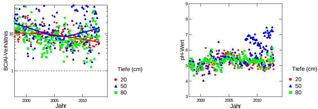
Abb. 329: Entwicklung des BC/Al-Verhältnisses (links) und des pH-Wertes (rechts) in der Bodenlösung der N-Versuchsfläche Zugerberg (ungedüngte Kontrollen).
