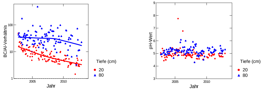
Abb. 273: Entwicklung des BC/Al-Verhältnisses (links) und des pH-Wertes (rechts) in der Bodenlösung der Buchenbeobachtungsfläche Rünenberg.
