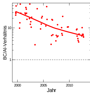
Abb. 177: Entwicklung des BC/Al-Verhältnisses (links) und des pH-Wertes (rechts) in der Bodenlösung der Fichtenbeobachtungsfläche Lurengo in 60 cm Bodentiefe.
