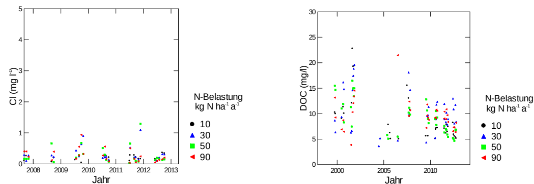
Abb. 364: Entwicklung der Chloridkonzentration (links) und der Konzentration an gelöstem organischen Kohlenstoff (rechts) in der Bodenlösung der N-Versuchsfläche Lurengo in 20 cm Tiefe
