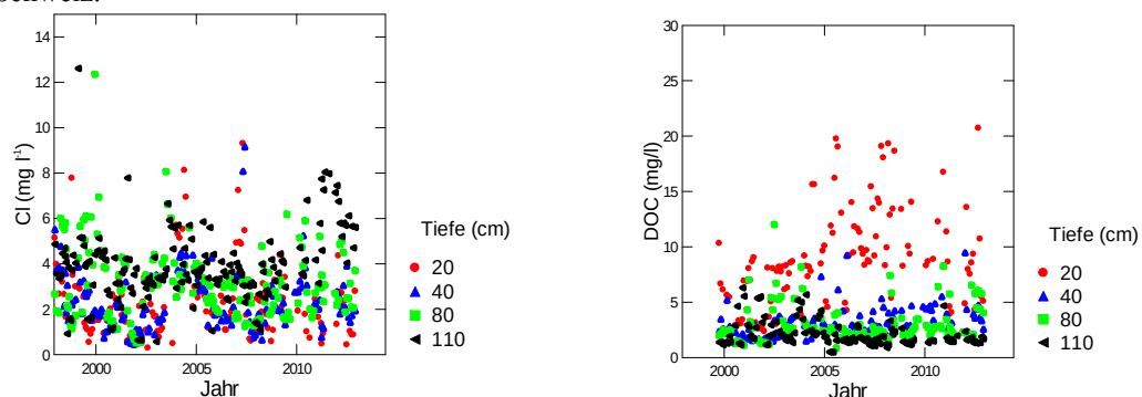
Abb. 108: Entwicklung der Chloridkonzentration (links) und der Konzentration an gelöstem organischen Kohlenstoff (rechts) in der Bodenlösung der Fichtenbeobachtungsfläche Brislach
