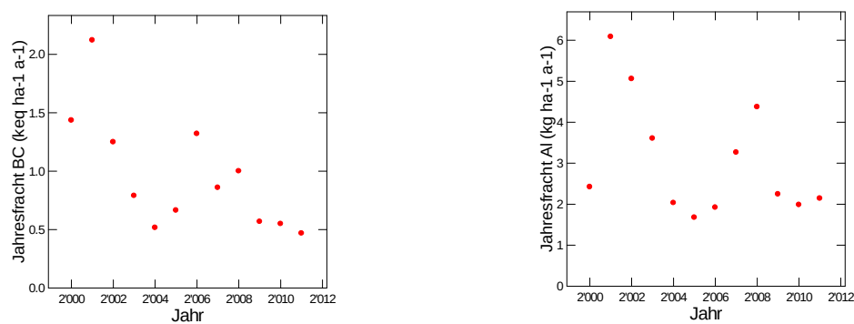
Abb. 223: Jährliche Frachten von basischen Kationen (links) und von Aluminium (rechts) in der Bodenlösung der Buchenbeobachtungsfläche Muri in 100 cm Tiefe.
