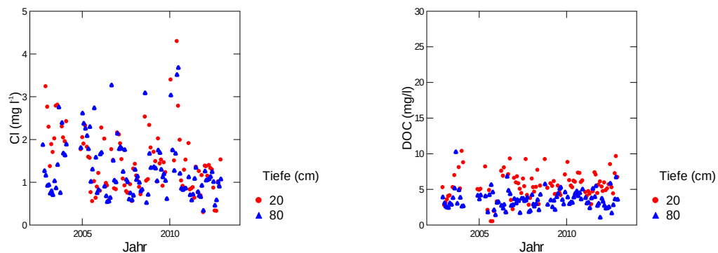
Abb. 164: Entwicklung der Chloridkonzentration (links) und der Konzentration an gelöstem organischen Kohlenstoff (rechts) in der Bodenlösung der Fichtenbeobachtungsfläche Hinwil.
