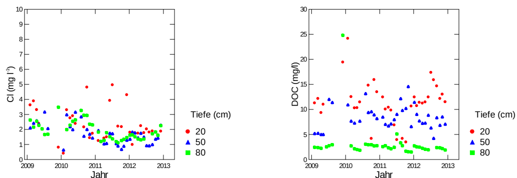
Abb. 300: Entwicklung der Chloridkonzentration (links) und der Konzentration an gelöstem organischem Kohlenstoff (rechts) in der Bodenlösung der Beobachtungsfläche Wangen
