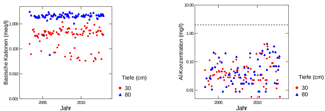
Abb. 98: Entwicklung der Konzentration von basischen Kationen (BC) (links) und der Konzentration von anorganischem Aluminium (rechts) in der Bodenlösung der Buchenbeobachtungsfläche Breitenbach. Die gestrichelte Linie in der rechten Grafik ist die kritische Al-Konzentration.
