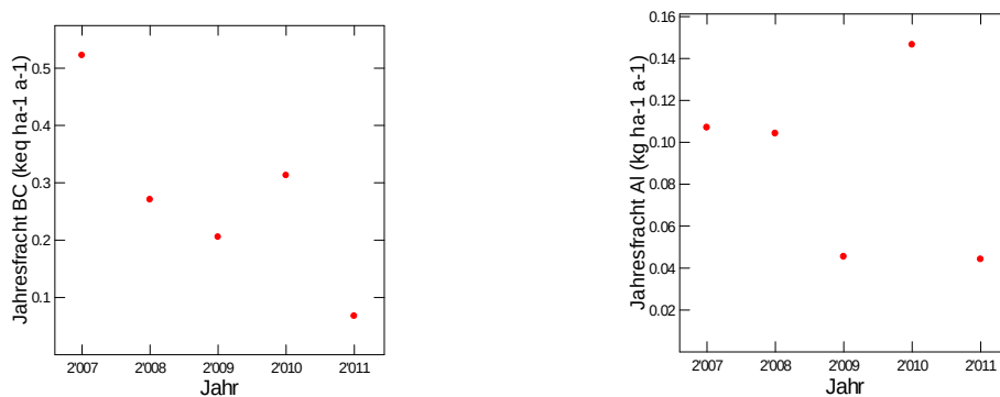
Abb. 239: Jährliche Frachten von basischen Kationen (links) und von Aluminium (rechts) in der Bodenlösung der Fichtenbeobachtungsfläche Oberschrot in 80 cm Tiefe.
