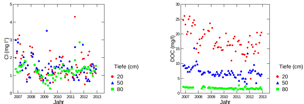
Abb. 132: Entwicklung der Chloridkonzentration (links) und der Konzentration an gelöstem organischen Kohlenstoff (rechts) in der Bodenlösung der Fichtenbeobachtungsfläche Diessenhofen.
