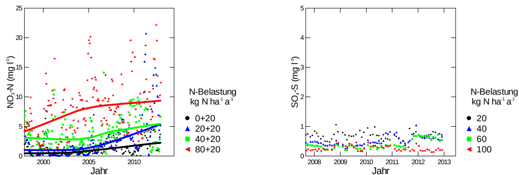
Abb. 355: Entwicklung der Konzentration von Nitratstickstoff (links) und von Sulfatschwefel (rechts) in der Bodenlösung der N-Versuchsfläche Zugerberg in 50 cm Tiefe
