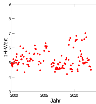
Abb. 281: Entwicklung des BC/Al-Verhältnisses (links) und des pH-Wertes (rechts) in der Bodenlösung der Fichtenbeobachtungsfläche Sagno in 60 cm Tiefe.
