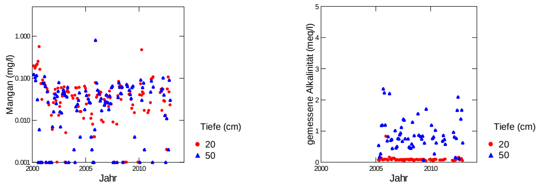
Abb. 117: Entwicklung der Mangankonzentration (links) und der gemessenen Alkalinität (rechts) in der Bodenlösung der Buchenbeobachtungsfläche Brislach
