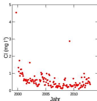
Abb. 220: Entwicklung der Chloridkonzentration (links) und der Konzentration an gelöstem organischem Kohlenstoff (rechts) in der Bodenlösung der Buchenbeobachtungsfläche Muri in 100 cm Bodentiefe.
