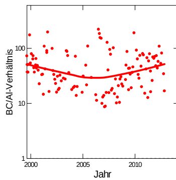
Abb. 281: Entwicklung des BC/Al-Verhältnisses (links) und des pH-Wertes (rechts) in der Bodenlösung der Fichtenbeobachtungsfläche Sagno in 60 cm Tiefe.
