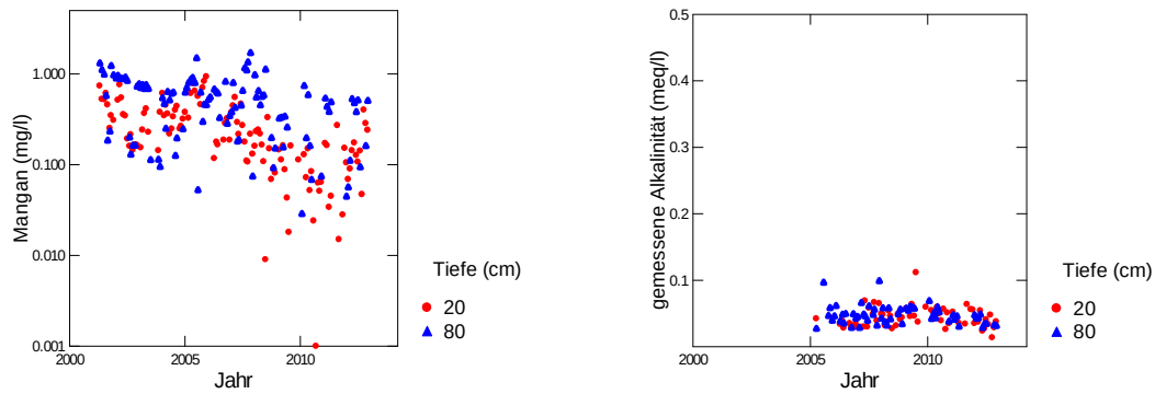
Abb. 157: Entwicklung der Mangankonzentration (links) und der gemessenen Alkalinität (rechts) in der Bodenlösung der Buchenbeobachtungsfläche Habsburg Kontrolle.
