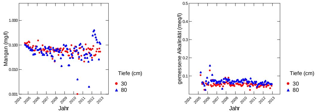
Abb. 125: Entwicklung der Mangankonzentration (links) und der gemessenen Alkalinität (rechts) in der Bodenlösung der Fichtenbeobachtungsfläche Busswil.
