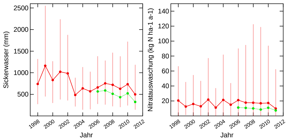
Abb. 20: Links Sickerwassermengen, rechts N-Auswaschung im seit mindestens 2001 beprobten Standortkollektiv. Dargestellt sind minimale, maximale und mittlere Jahressummen (n=12). Benachbarte Flächen wurden für diese Auswertung zusammengefasst, um eine regionale Überrepräsentierung zu vermeiden. Grüne Linie: alle Flächen mit Messung seit mindestens 2006 (n=31).
