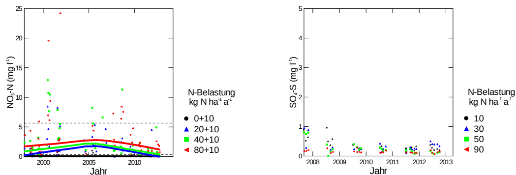
Abb. 363: Entwicklung der Konzentration von Nitratstickstoff (links) und von Sulfatschwefel (rechts) in der Bodenlösung der N-Versuchsfläche Lurengo in 20 cm Tiefe
