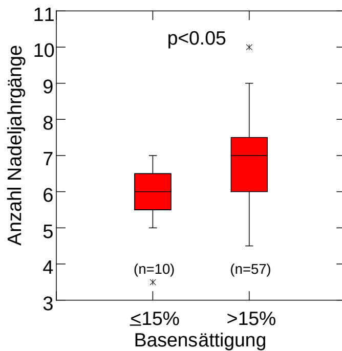
Abb. 14: Anzahl Nadeljahrgänge bei den Fichten in Beziehung zur über die obersten 40 cm gemittelten Basensättigung des Bodens. n: Anzahl Flächen (8 Bäume pro Fläche).
