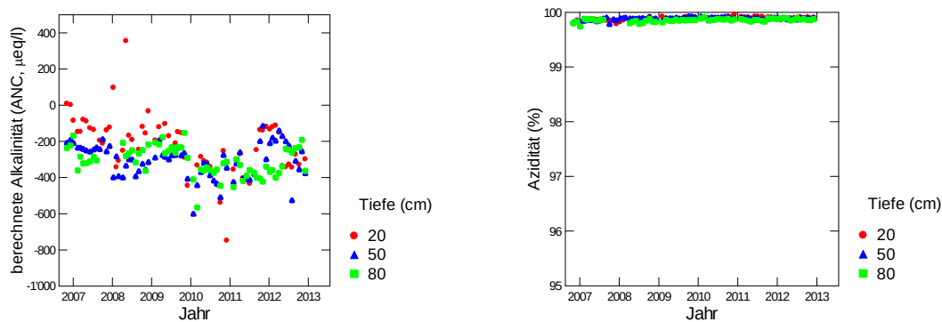
Abb. 134: Entwicklung der berechneten Alkalinität (links) und der Azidität (rechts) in der Bodenlösung der Fichtenbeobachtungsfläche Diessenhofen.
