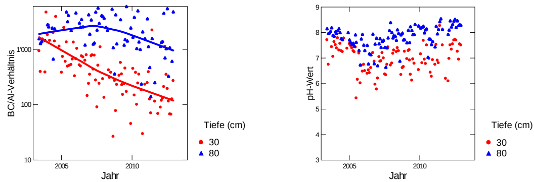
Abb. 313: Entwicklung des BC/Al-Verhältnisses (links) und des pH-Wertes (rechts) in der Bodenlösung der Fichtenbeobachtungsfläche Winterthur.
