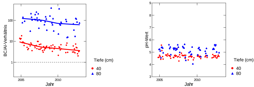
Abb. 225: Entwicklung des BC/Al-Verhältnisses (links) und des pH-Wertes (rechts) in der Bodenlösung der Buchenbeobachtungsfläche Muttenz.
