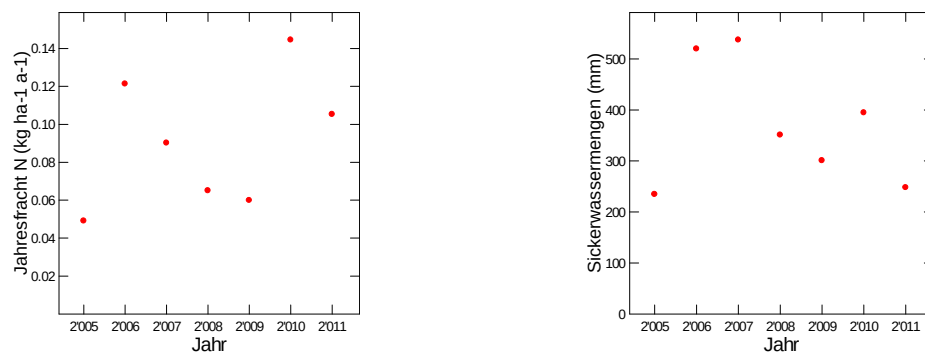
Abb. 128: Jährliche N-Fracht (links) und Sickerwassermenge (rechts) in der Bodenlösung der Fichtenbeobachtungsfläche Busswil in 80 cm Tiefe.
