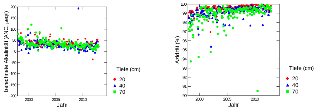
Abb. 310: Entwicklung der berechneten Alkalinität (links) und der Azidität (rechts) in der Bodenlösung der Fichtenbeobachtungsfläche Wengernalp.
