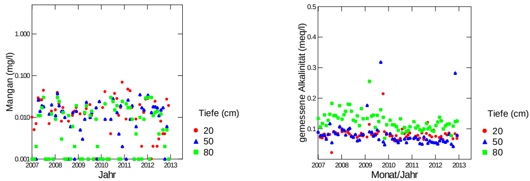
Abb. 173: Entwicklung der Mangankonzentration (links) und der gemessenen Alkalinität (rechts) in der Bodenlösung der Fichtenbeobachtungsfläche Le Châtelard.
