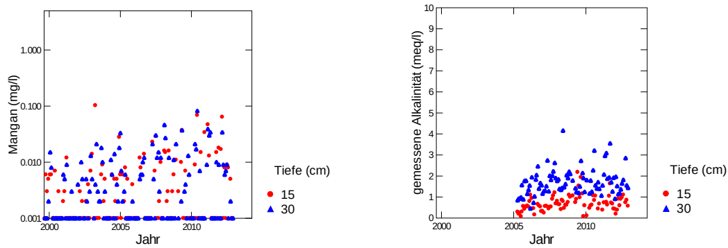
Abb. 149: Entwicklung der Mangankonzentration (links) und der gemessenen Alkalinität (rechts) in der Bodenlösung der Beobachtungsfläche Grenchenberg (Buchen/Fichten).
