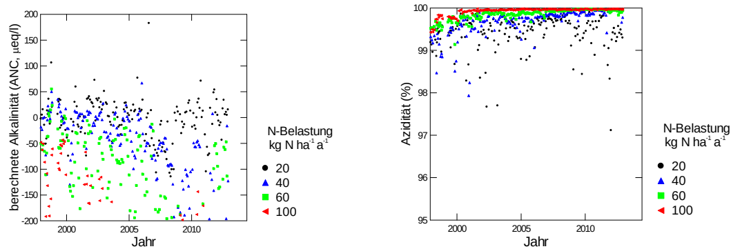
Abb. 358: Entwicklung der berechneten Alkalinität (links) und der Azidität (rechts) in der Bodenlösung der N-Versuchsfläche Zugerberg in 50 cm Tiefe.
