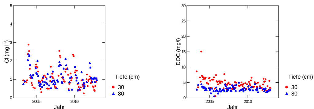
Abb. 100: Entwicklung der Chloridkonzentration (links) und der Konzentration an gelöstem organischen Kohlenstoff (rechts) in der Bodenlösung der Buchenbeobachtungsfläche Breitenbach.
