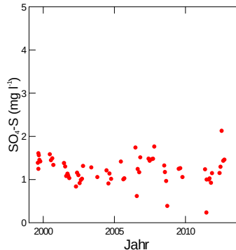
Abb. 179: Entwicklung der Konzentration von Nitratstickstoff (links) und von Sulfatschwefel (rechts) in der Bodenlösung der Fichtenbeobachtungsfläche Lurengo in 60 cm Bodentiefe. In der linken Grafik entspricht die untere gestrichelte Linie der maximal zulässigen N-Auswaschung, die obere Linie dem Nitrat-Qualitätsziel für Trinkwasser in der Schweiz.
