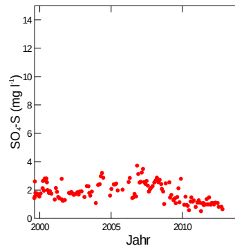
Abb. 283: Entwicklung der Konzentration von Nitratstickstoff (links) und von Sulfatschwefel (rechts) in der Bodenlösung der Fichtenbeobachtungsfläche Sagno in 60 cm Tiefe. In der linken Grafik entspricht die untere gestrichelte Linie der maximal zulässigen N-Auswaschung, die obere Linie dem Nitrat-Qualitätsziel für Trinkwasser in der Schweiz.
