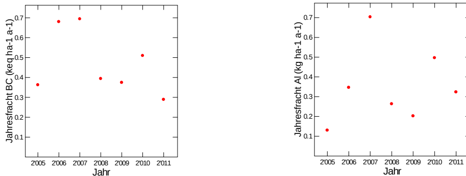
Abb. 127: Jährliche Frachten von basischen Kationen (links) und von Aluminium (rechts) in der Bodenlösung der Fichtenbeobachtungsfläche Busswil in 80 cm Tiefe.
