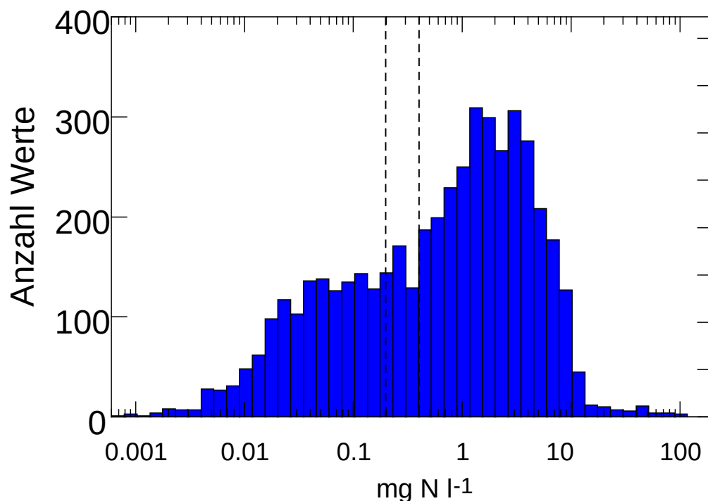
Abb. 16: Häufigkeitsverteilung der Konzentration an anorganischem Stickstoff in der Bodenlösung in <70 cm Tiefe ( \text{NO}_3^- + \text{NH}_4^+ ) zwischen 2005 und 2011 (einzelne Monatswerte). Eingetragen ist der Grenzwertbereich für Konzentrationen bezüglich Nährstoffungleichgewichten (Tab. 3)
