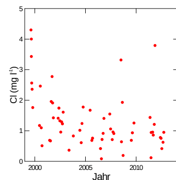
Abb. 180: Entwicklung der Chloridkonzentration (links) und der Konzentration an gelöstem organischem Kohlenstoff (rechts) in der Bodenlösung der Fichtenbeobachtungsfläche Lurengo in 60 cm Bodentiefe.
