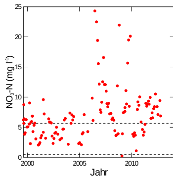
Abb. 283: Entwicklung der Konzentration von Nitratstickstoff (links) und von Sulfatschwefel (rechts) in der Bodenlösung der Fichtenbeobachtungsfläche Sagno in 60 cm Tiefe. In der linken Grafik entspricht die untere gestrichelte Linie der maximal zulässigen N-Auswaschung, die obere Linie dem Nitrat-Qualitätsziel für Trinkwasser in der Schweiz.
