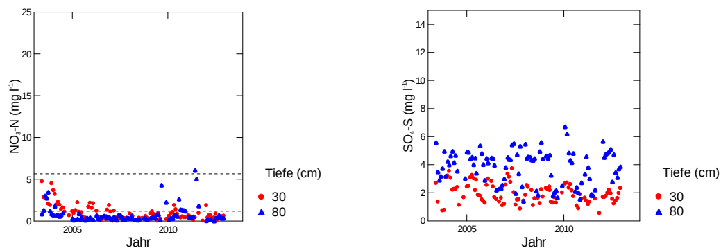
Abb. 315: Entwicklung der Konzentration von Nitratstickstoff (links) und von Sulfatschwefel (rechts) in der Bodenlösung der Fichtenbeobachtungsfläche Winterthur. In der linken Grafik entspricht die untere gestrichelte Linie der maximal zulässigen N-Auswaschung, die obere Linie dem Nitrat-Qualitätsziel für Trinkwasser in der Schweiz.
