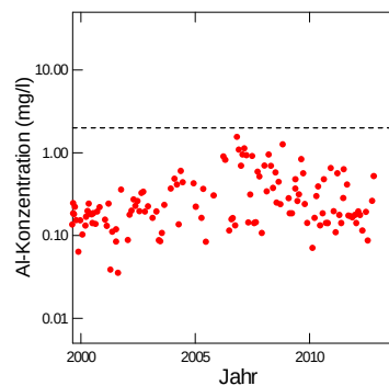
Abb. 282: Entwicklung der Konzentration von basischen Kationen (BC) (links) und der Konzentration von anorganischem Aluminium (rechts) in der Bodenlösung der Fichtenbeobachtungsfläche Sagno in 60 cm Tiefe. Die gestrichelte Linie in der rechten Grafik ist die kritische Al-Konzentration.
