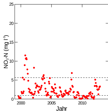
Abb. 219: Entwicklung der Konzentration von Nitratstickstoff (links) und von Sulfatschwefel (rechts) in der Bodenlösung der Buchenbeobachtungsfläche Muri in 100 cm Bodentiefe. In der linken Grafik entspricht die untere gestrichelte Linie der maximal zulässigen N-Auswaschung, die obere Linie dem Nitrat-Qualitätsziel für Trinkwasser in der Schweiz.
