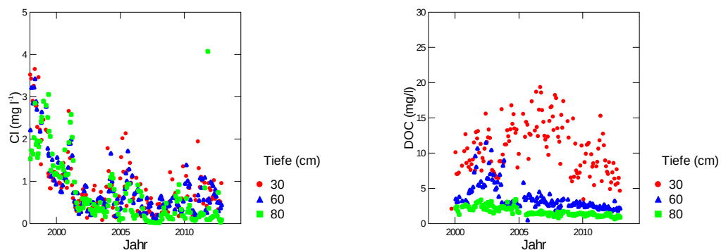
Abb. 204: Entwicklung der Chloridkonzentration (links) und der Konzentration an gelöstem organischen Kohlenstoff (rechts) in der Bodenlösung der (ehemaligen) Fichtenbeobachtungsfläche Muri.
