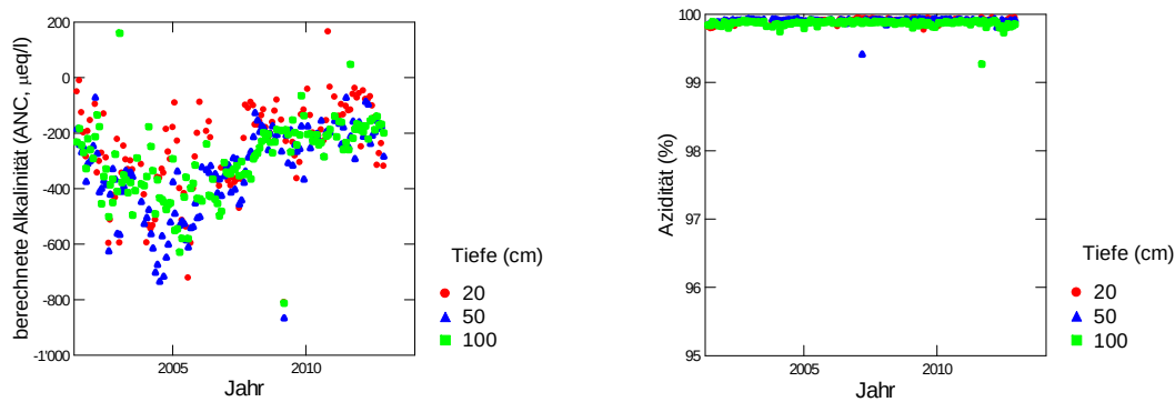
Abb. 214: Entwicklung der berechneten Alkalinität (links) und der Azidität (rechts) in der Bodenlösung der neuen Fichtenbeobachtungsfläche Muri.
