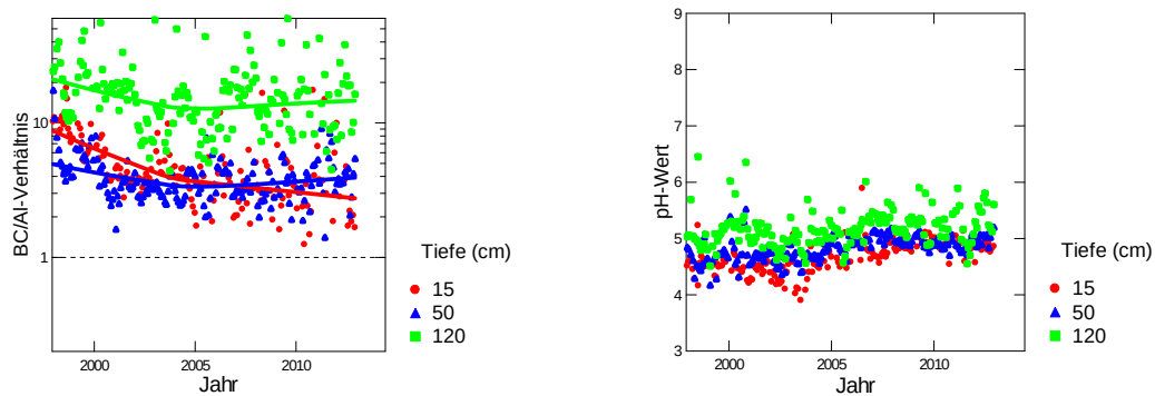
Abb. 137 Entwicklung des BC/Al-Verhältnisses (links) und des pH-Wertes (rechts) in der Bodenlösung der Beobachtungsfläche Frienisberg (Mischbestand Buchen/Fichten).
