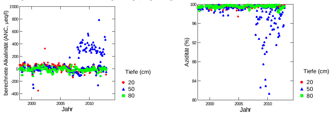
Abb. 334: Entwicklung der berechneten Alkalinität (links) und der Azidität (rechts) in der Bodenlösung der N-Versuchsfläche Zugerberg (ungedüngte Kontrollen).
