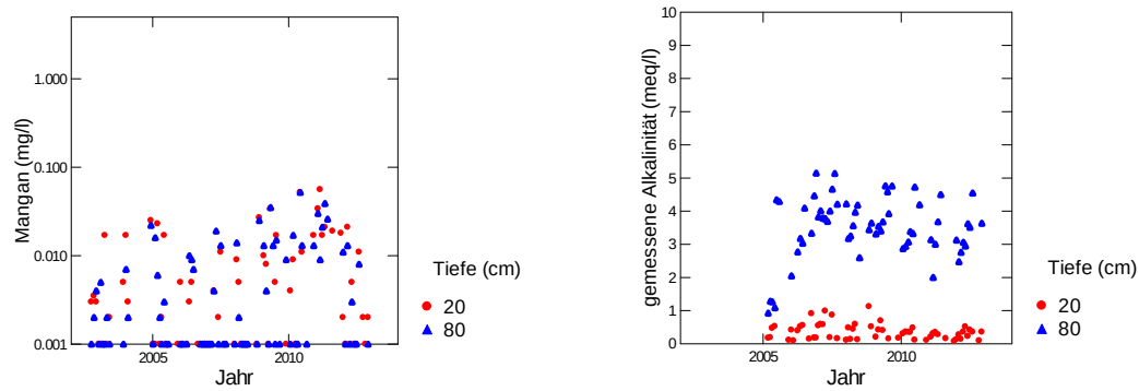
Abb. 253: Entwicklung der Mangankonzentration (links) und der gemessenen Alkalinität (rechts) in der Bodenlösung der Buchenbeobachtungsfläche Pratteln.
