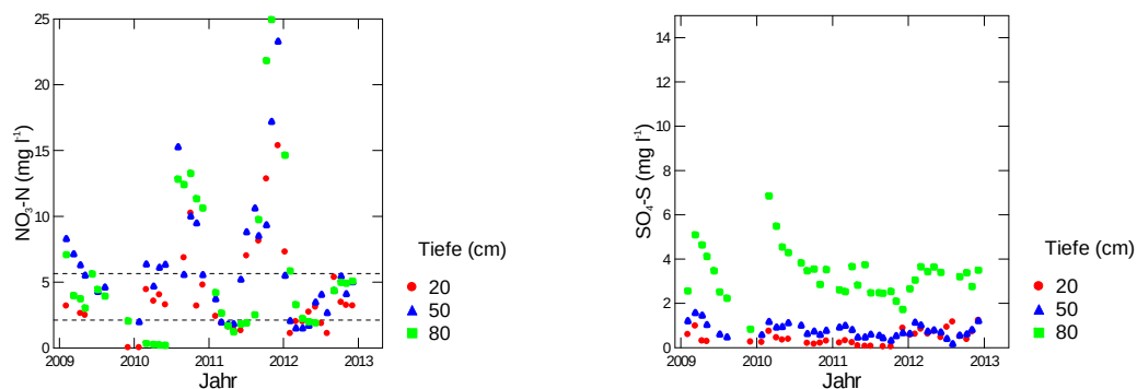
Abb. 299: Entwicklung der Konzentration von Nitratstickstoff (links) und von Sulfatschwefel (rechts) in der Bodenlösung der Beobachtungsfläche Wangen. In der linken Grafik entspricht die untere gestrichelte Linie der maximal zulässigen N-Auswaschung, die obere Linie dem Nitrat-Qualitätsziel für Trinkwasser in der Schweiz.
