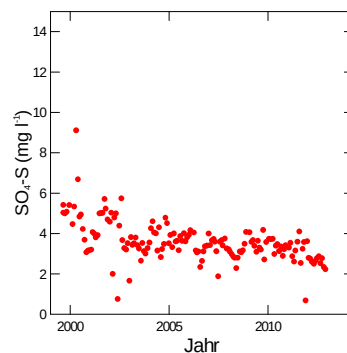
Abb. 219: Entwicklung der Konzentration von Nitratstickstoff (links) und von Sulfatschwefel (rechts) in der Bodenlösung der Buchenbeobachtungsfläche Muri in 100 cm Bodentiefe. In der linken Grafik entspricht die untere gestrichelte Linie der maximal zulässigen N-Auswaschung, die obere Linie dem Nitrat-Qualitätsziel für Trinkwasser in der Schweiz.
