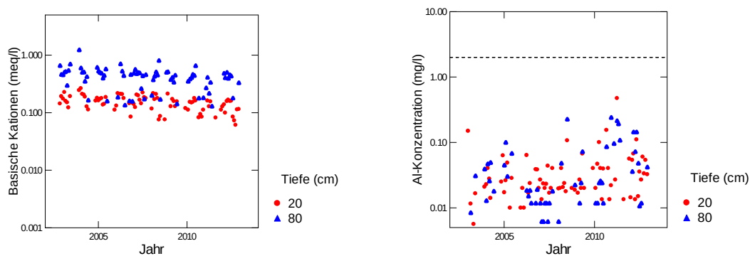
Abb. 266: Entwicklung der Konzentration von basischen Kationen (BC) (links) und der Konzentration von anorganischem Aluminium (rechts) in der Bodenlösung der Buchenbeobachtungsfläche Riehen Mittelberg. Die gestrichelte Linie in der rechten Grafik ist die kritische Al-Konzentration.
