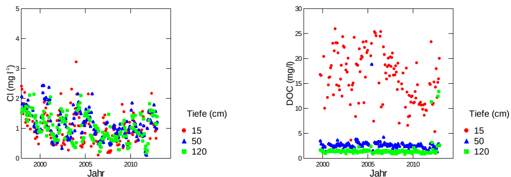
Abb. 140: Entwicklung der Chloridkonzentration (links) und der Konzentration an gelöstem organischen Kohlenstoff (rechts) in der Bodenlösung der Beobachtungsfläche Frienisberg
