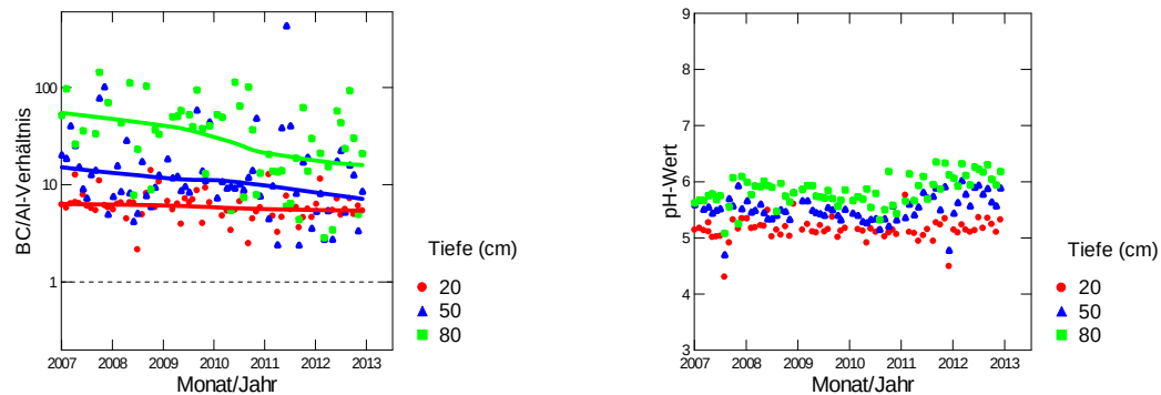
Abb. 233: Entwicklung des BC/Al-Verhältnisses (links) und des pH-Wertes (rechts) in der Bodenlösung der Fichtenbeobachtungsfläche Oberschrot.
