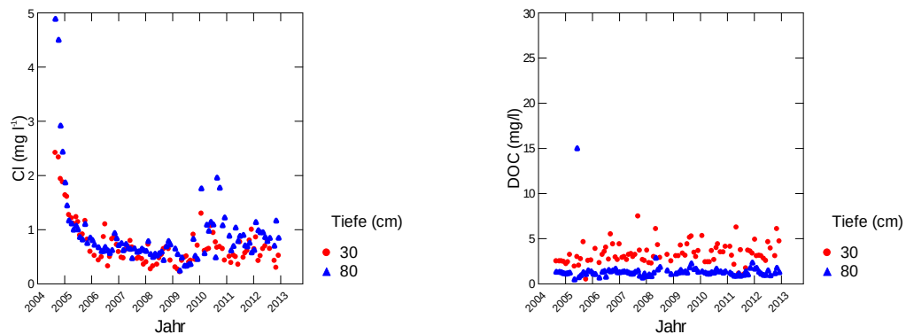
Abb. 124: Entwicklung der Chloridkonzentration (links) und der Konzentration an gelöstem organischen Kohlenstoff (rechts) in der Bodenlösung der Fichtenbeobachtungsfläche Busswil.
