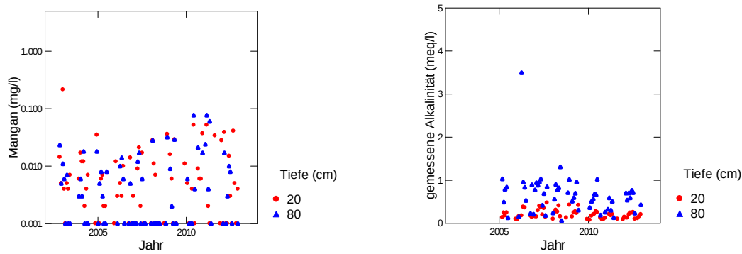
Abb. 269: Entwicklung der Mangankonzentration (links) und der gemessenen Alkalinität (rechts) in der Bodenlösung der Buchenbeobachtungsfläche Riehen Mittelberg.
