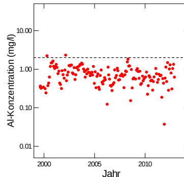
Abb. 218: Entwicklung der Konzentration von basischen Kationen (BC) (links) und der Konzentration von anorganischem Aluminium (rechts) in der Bodenlösung der Buchenbeobachtungsfläche Muri in 100 cm Bodentiefe. Die gestrichelte Linie in der rechten Grafik ist die kritische Al-Konzentration.
