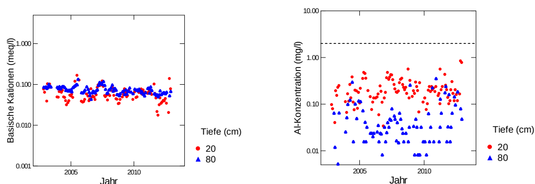
Abb. 34: Entwicklung der Konzentration von basischen Kationen (BC) (links) und der Konzentration von anorganischem Aluminium (rechts) in der Bodenlösung der Buchenbeobachtungsfläche Aarwangen. Die gestrichelte Linie in der rechten Grafik ist die kritische Al-Konzentration.
