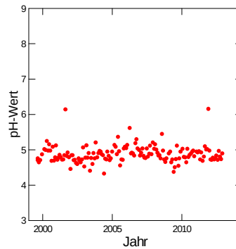
Abb. 217: Entwicklung des BC/Al-Verhältnisses (links) und des pH-Wertes (rechts) in der Bodenlösung der Buchenbeobachtungsfläche Muri in 100 cm Bodentiefe. Die Lysimeter in einer Tiefe von 20 cm wurden 2006 neu installiert.
